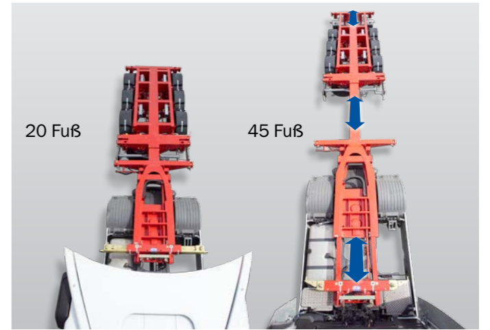
Teleskopierung des Vario Chassis
