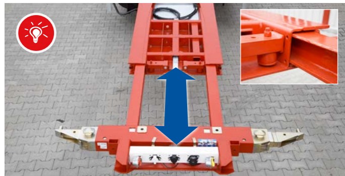
Rollengelagerter, gummigedämpfter Frontausschub für mehr Langlebigkeit und komfortables Handling
